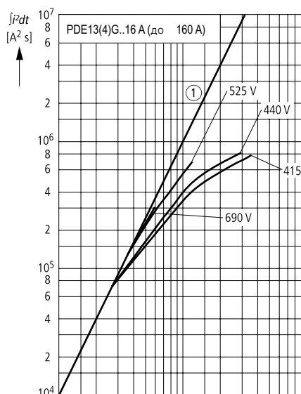
Пропускаемая энергия I^2t ; PDE1 TMTU PDE13(4)G..16 A (до 160 A)
