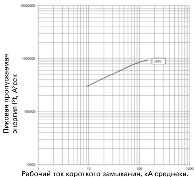
Пропускаемая энергия I^2t ; PDE2 ETU PXR10 LSI; 100 А и 160 А при 240 В
