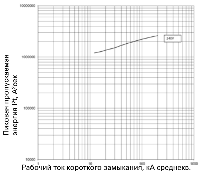
Пропускаемая энергия I^2t ; PDE3 ETU PXR10 LI; 400 А при 240 В
