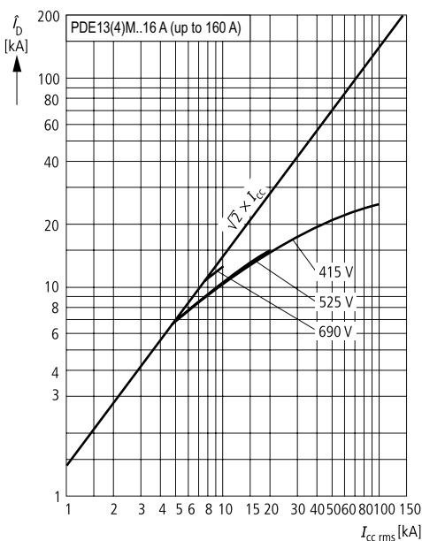
Сквозной ток ID PDE1 TMTU PDE13(4)M..16 A (до 160 A)
