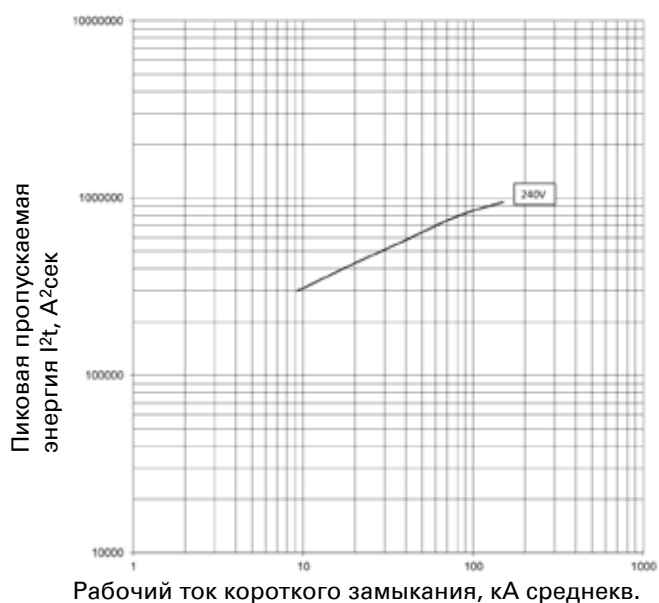
Пропускаемая энергия I^2t ; PDE9 ETU PXR10 LI; 63 А и 100 А при 240 В
