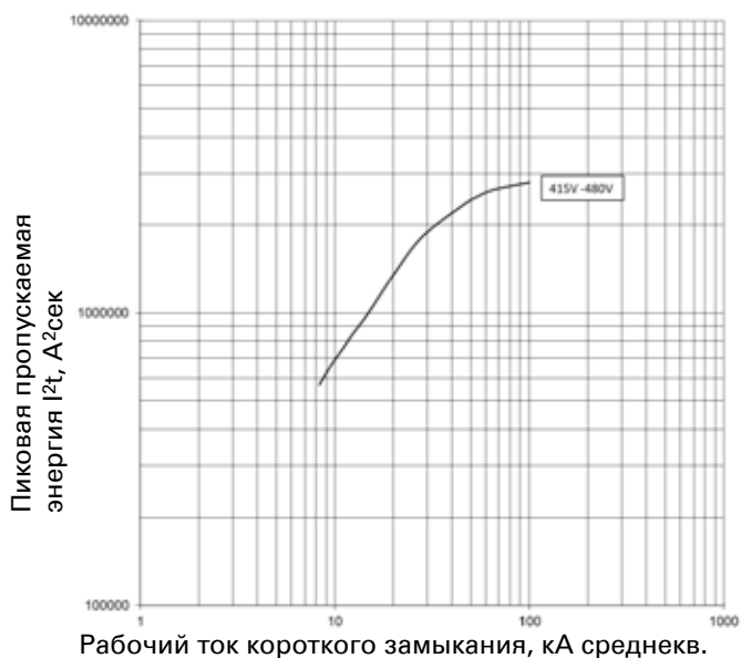
Пропускаемая энергия I^2t ; PDE2 ETU PXR10 LI; 160 А при 415 В и 440 В
