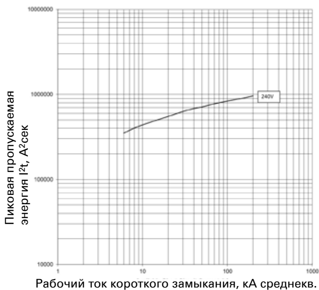
Пропускаемая энергия I^2t ; PDE2 ETU PXR10 LI; 200 А при 415 В и 440 В
