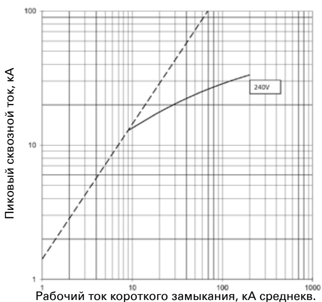
Сквозной ток I_D PDE2 TMTU; 200 A при 240 В
