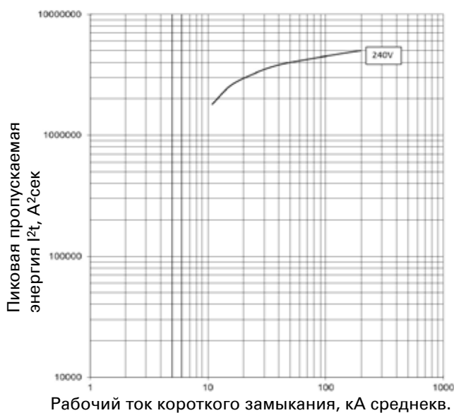
Пропускаемая энергия I^2t ; PDE3 ETU PXR10 LI; 630 А при 240 В
