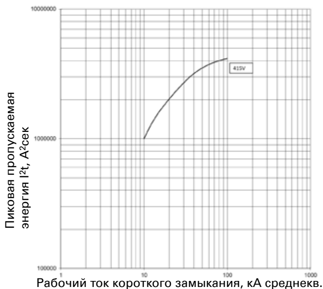
Пропускаемая энергия I^2t ; PDE3 ETU PXR10 LI; 400 А при 415 В
