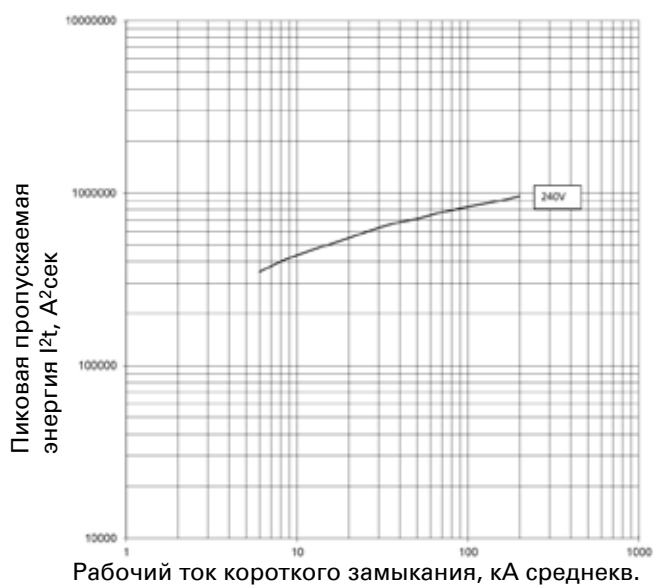
Пропускаемая энергия I^2t ; PDE2 ETU PXR10 LI; 200 А при 240 В
