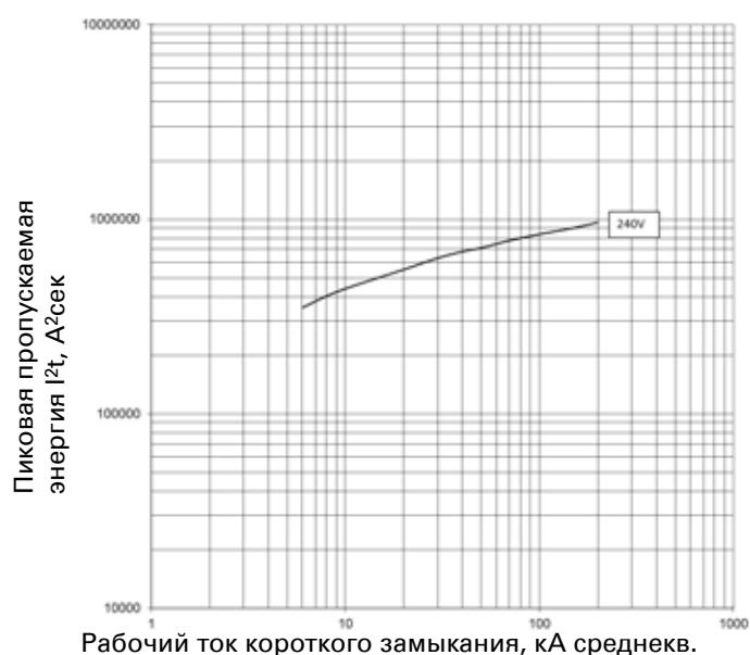
Пропускаемая энергия I^2t ; PDE2 ETU PXR10 LSI; 220 А при 415 В и 440 В
