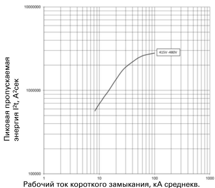
Пропускаемая энергия I^2t ; PDE9 ETU PXR10 LI; 63 А и 100 А при 415 В и 440 В
