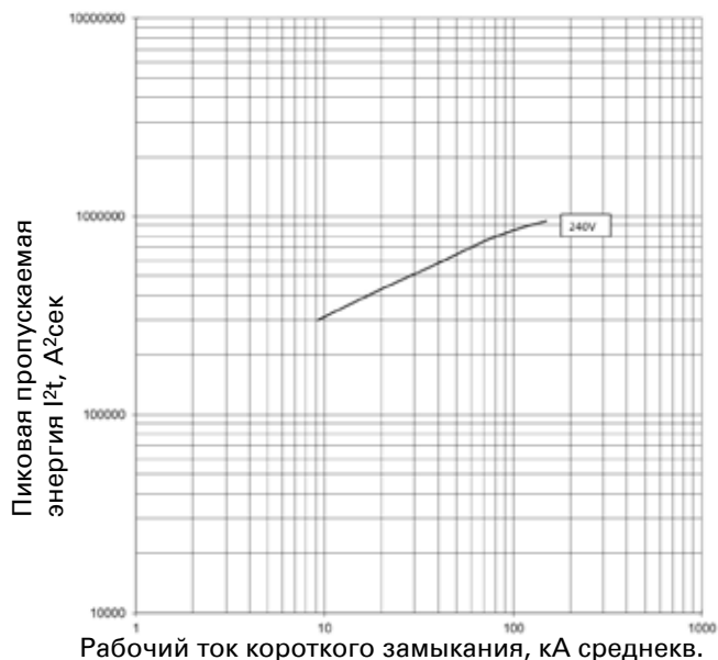
Пропускаемая энергия I^2t ; PDE2 ETU PXR10 LI; 160 А при 240 В
