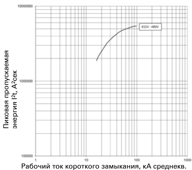
Пропускаемая энергия I^2t ; PDE3 ETU PXR10 LI; 400 А при 440 В
