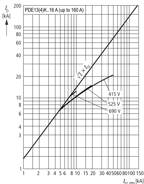
Сквозной ток ID PDE1 TMTU PDE13(4)K..16 A (до 160 A)
