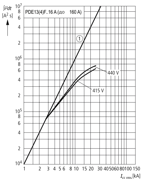
Пропускаемая энергия I^2t ; PDE1 TMTU PDE13(4)F..16 A (до 160 A)
