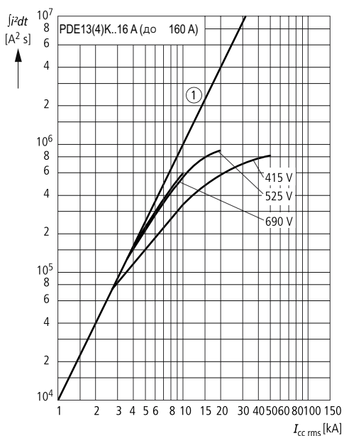
Пропускаемая энергия I^2t ; PDE1 TMTU PDE13(4)K..16 A (до 160 A)
