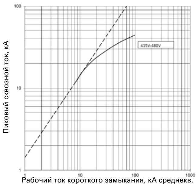
Сквозной ток I_D PDE2 TMTU; 200 A при 415 В и 440 В
