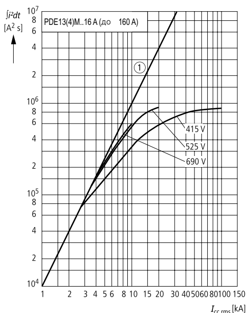
Пропускаемая энергия I^2t ; PDE1 TMTU PDE13(4)M..16 A (до 160 A)
