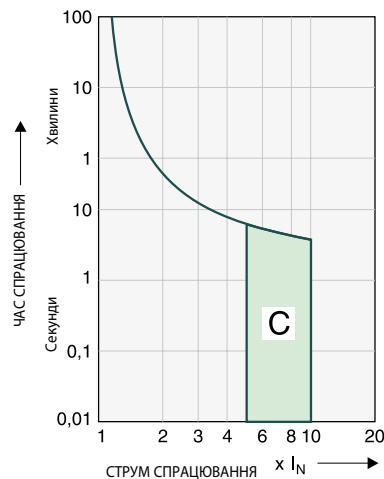
Характеристика спрацювання С
