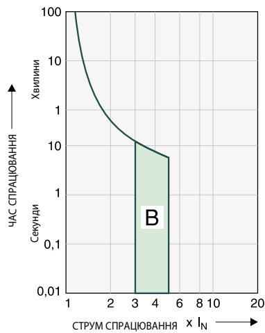
Характеристика спрацювання В
