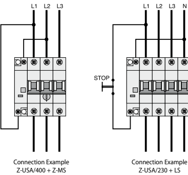
Приклад приєднання 400В і 230В
