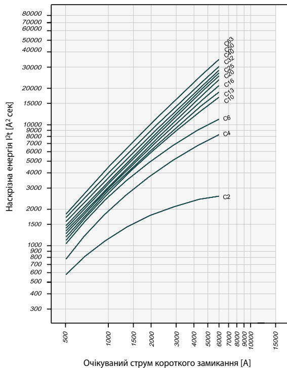
Наскрізна енергія PL6, Характеристика С, 1-полюс
